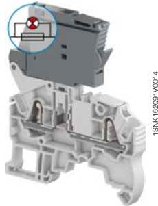
ZK2.5-SF-R
